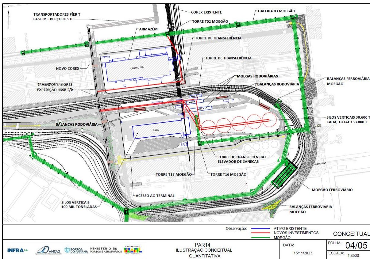
Figura 02: Layout conceitual da área de arrendamento PAR14 – Porto de Paranaguá/PR.
